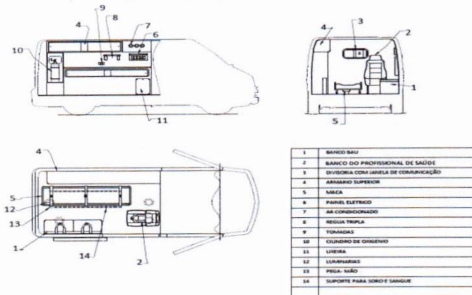
Foto 1: Disposição de oxigênio e 1 de Ar ambulâncias do tipo B
